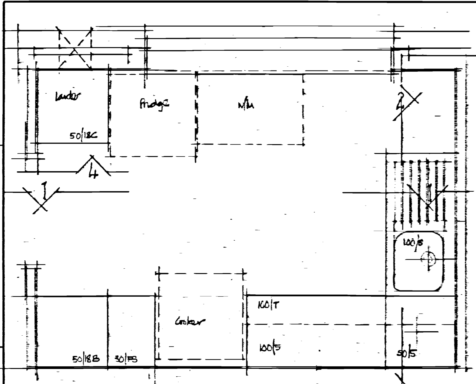
BEDSITTER LAYOUT
